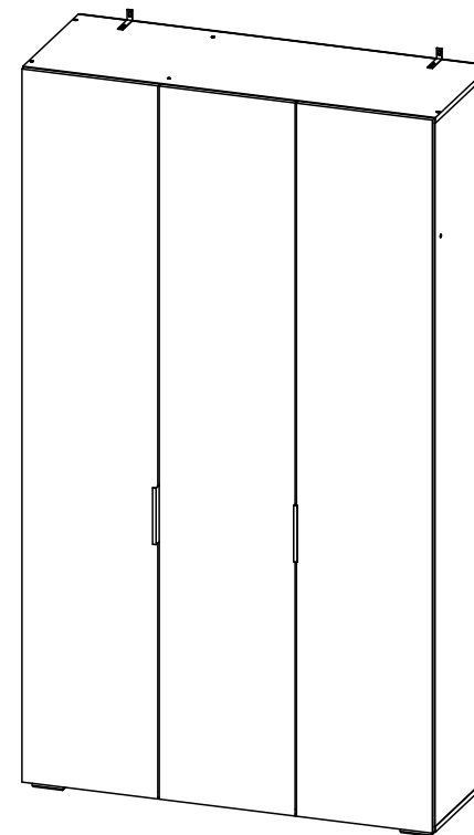
«Соната» ШК-03 Шкаф 3х-створчатый ↔ 1200 ↑ 2100 ↗ 460 «Sonata» Shk-03 3-fold cabinet
